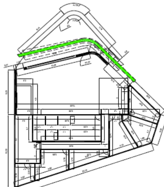
PLANTA DE COTAS
