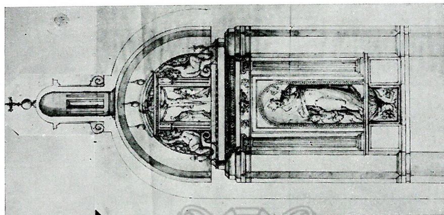
Esquema de la traza del hueco y arco de la capilla de los Moyas, en Santa María Magdalena, dibujados por Alonso de Barba, cuya firma aparece al pie. A la derecha, dibujo del retablo de la capilla hecho por el entallador de Jaén, Sebastián de Solís
